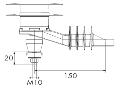
Odłącznik uziemienia z podstawą izolacyjną
