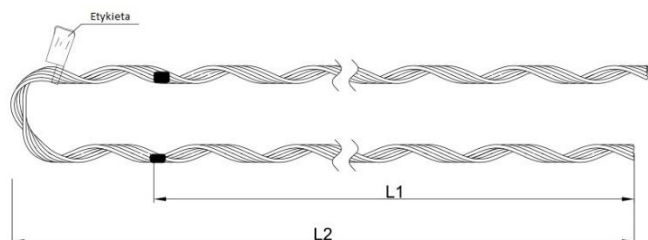
PĘTLA OTWARTA
