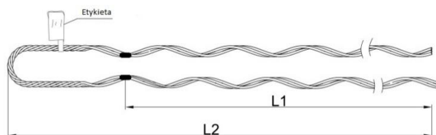
PĘTLA SKRĘCONA
